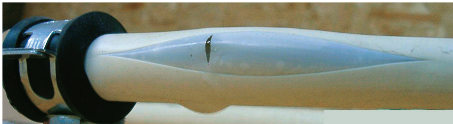
Névlegesnél kisebb nyomáson felhasadt csővezeték
