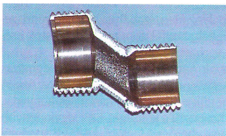
Papírvékony falú Z-idom
